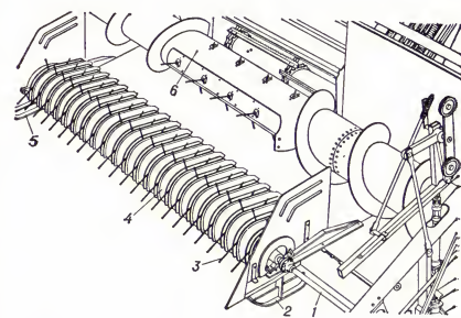
Рис. 1. Подборщик барабанного типа: 1 — приводной вал; 2 и 5 — опорные башмаки; 3 — пружинные пальцы; 4 — цилиндрический кожух; 6 — пневматический транспортёр жатки комбайна.
